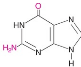
Guanine (G) (2-amino 6-oxypurine)
